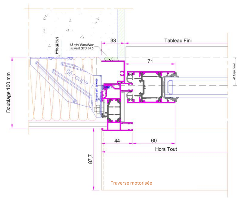
Montant latéral ALU – doublage 100
