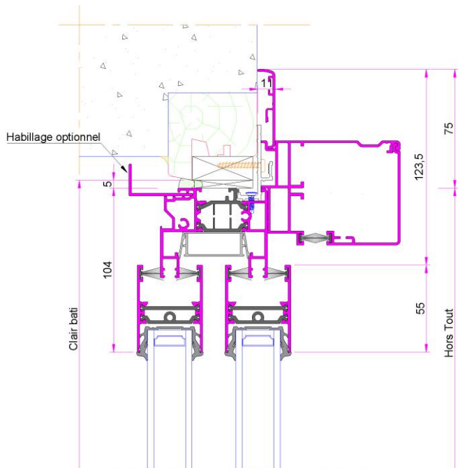
Traverse Haute ALU
