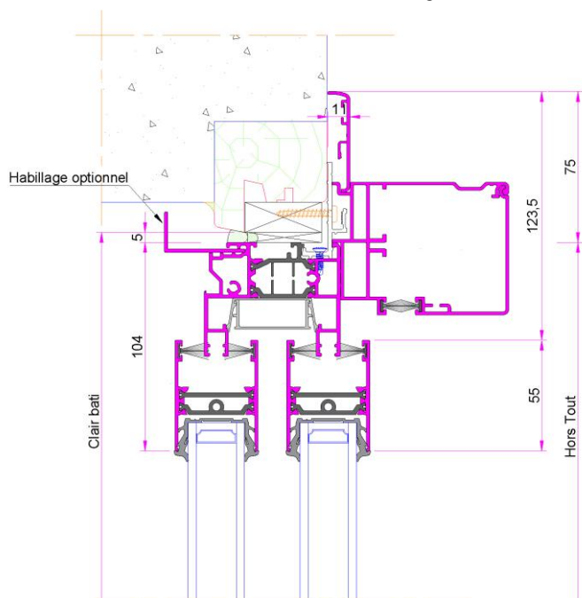
Traverse Haute ALU – doublage 100
