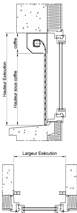
Pose en tableau Enroulement extérieur
