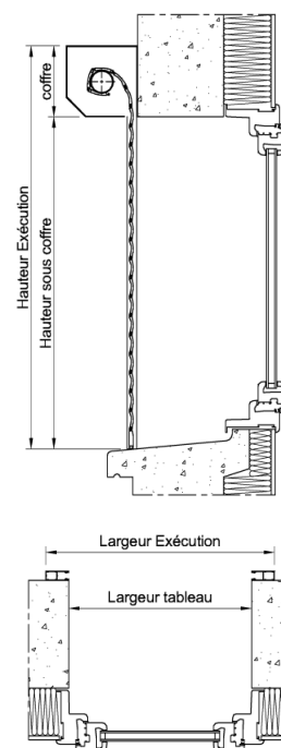
Pose en applique Enroulement extérieur
