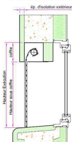
Pose en tableau Enroulement intérieur
