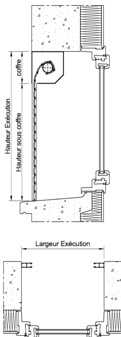
Pose en tableau Enroulement intérieur
