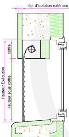
Pose en tableau Enroulement intérieur
