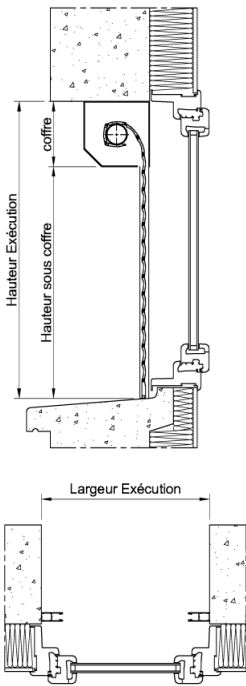
Pose en tableau Enroulement extérieur
