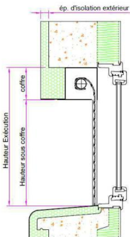
Pose en tableau Enroulement extérieur
