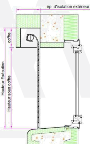
Pose en applique Enroulement extérieur
