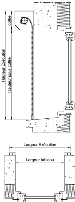
Pose en applique Enroulement extérieur
