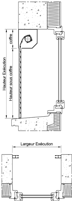
Pose en tableau Enroulement intérieur
