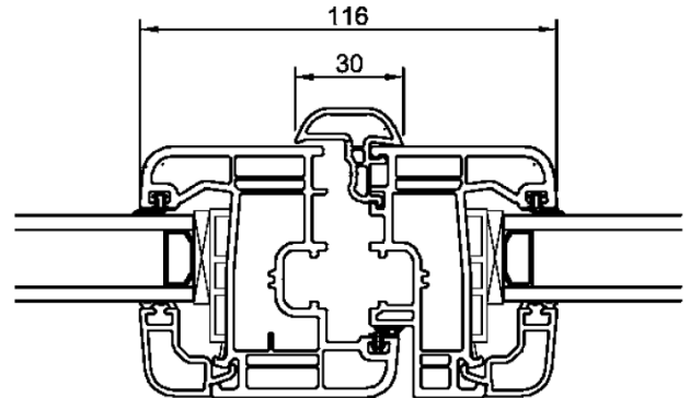
Battements avec profil d'ouvrant FENETRE
