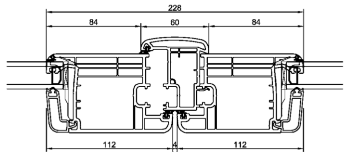
Battements avec profil d'ouvrant PORTE D'ENTREE Ouverture intérieure
