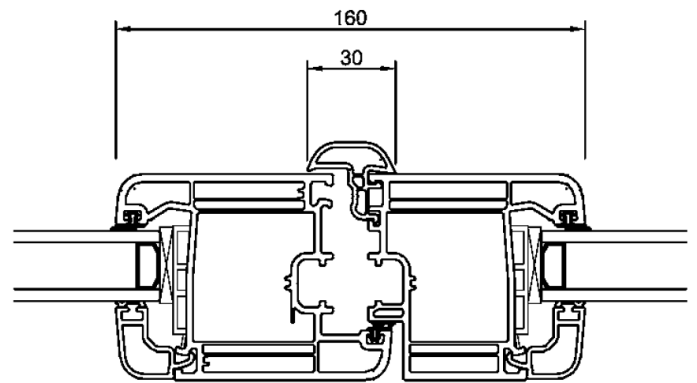
Battements avec profil d'ouvrant PORTE FENETRE
