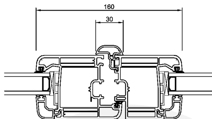
Battements avec profil d'ouvrant PORTE FENETRE
