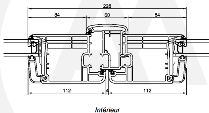
Battements avec profil d'ouvrant PORTE D'ENTREE Ouverture intérieure
