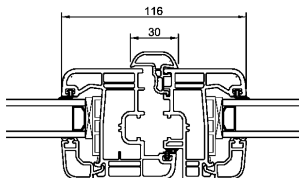
Battements avec profil d'ouvrant FENETRE
