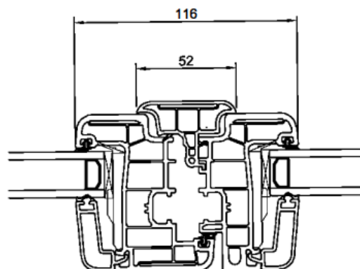
Battements avec profil d'ouvrant FENETRE
