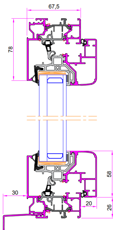
Coupe verticale OF 2 dormant de base – vitrage de 34 mm
