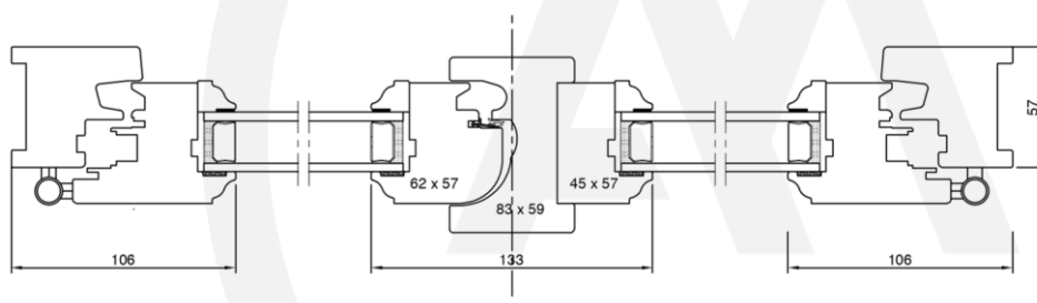
Coupe horizontale OF 2 dormant de base, battement central Mouton et Gueule de Loup
